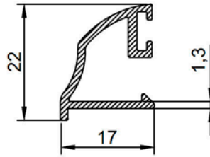
ER 7210 0,228 kg/m 24 mm Boşluklu Cam Çıtası Glazing With 24 mm Gap
