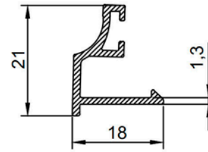
ER 7211 0,190 kg/m 30 mm Boşluklu Cam Çıtası Glazing With 30 mm Gap
