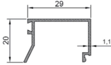
ER 1630 0,219 kg/m Tek Cam Çıta Profili Single Glazing Bead Profile
